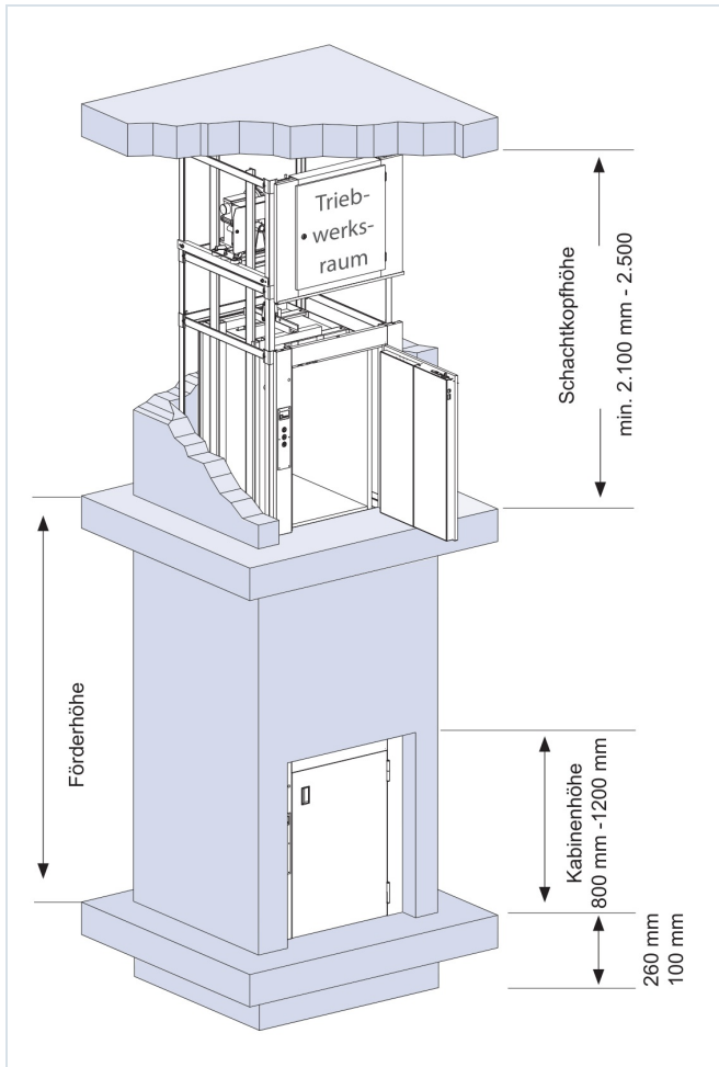
Schematische Darstellung „CARGO Line“ mit Drehtüren, Bodengleich. Zugänge / Beladung von max. 3 Seiten möglich.
