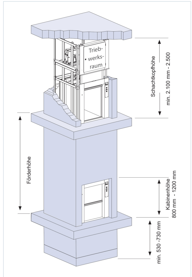
Schematische Darstellung „CARGO Line“ mit Schiebetüren, Bodengleich. Zugänge / Beladung von max. 3 Seiten möglich.
